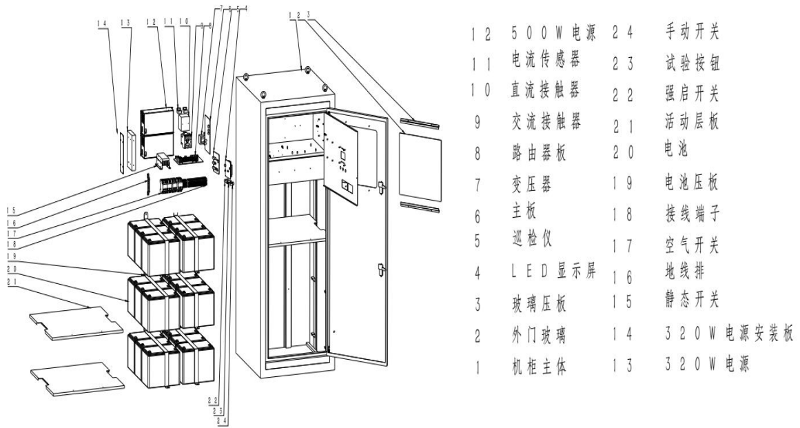
图 2 结构图
