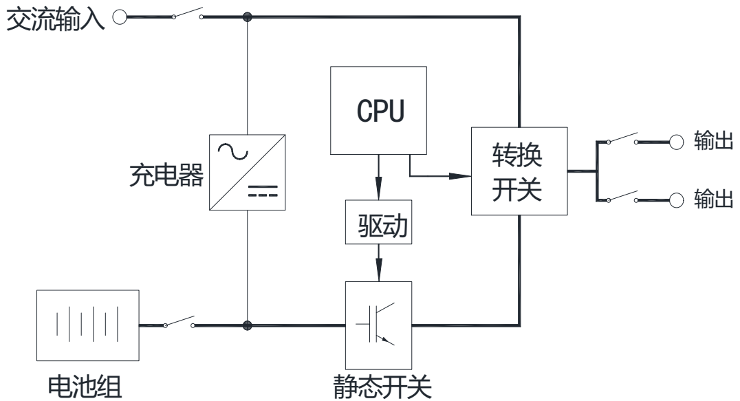
图 3 工作原理图
