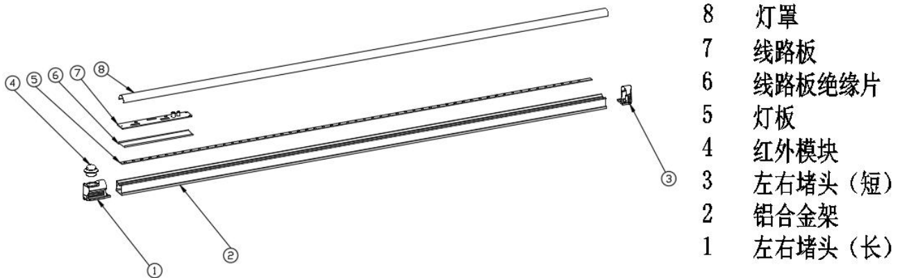
图 2 T8-18H 型结构示意图
