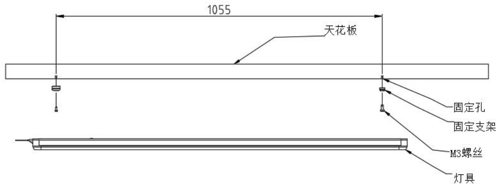
图 4 T8-18H 安装示意图
